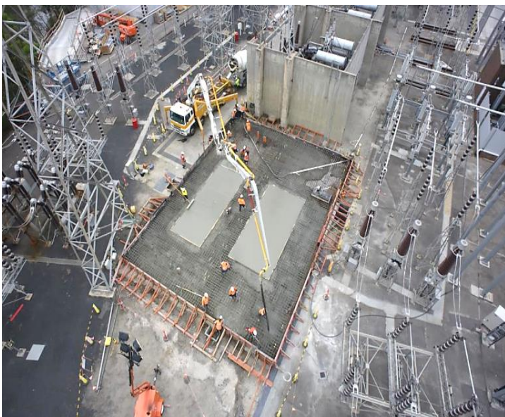
Concrete Pour for Transformer Slab
