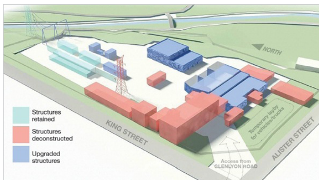
Σχηματικό διάγραμμα της αναβάθμισης του Τερματικού Σταθμού στο Brunswick
